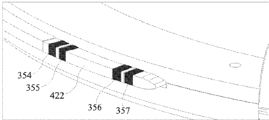
FIG. 33
